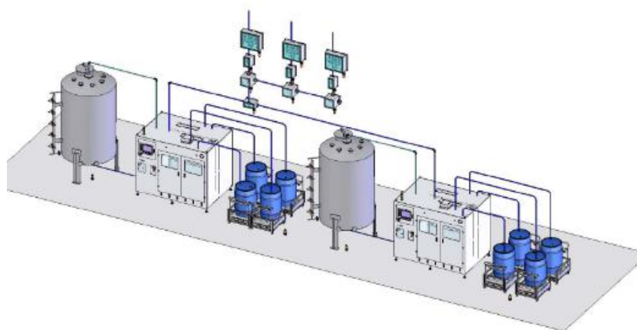
(高纯特气柜)
